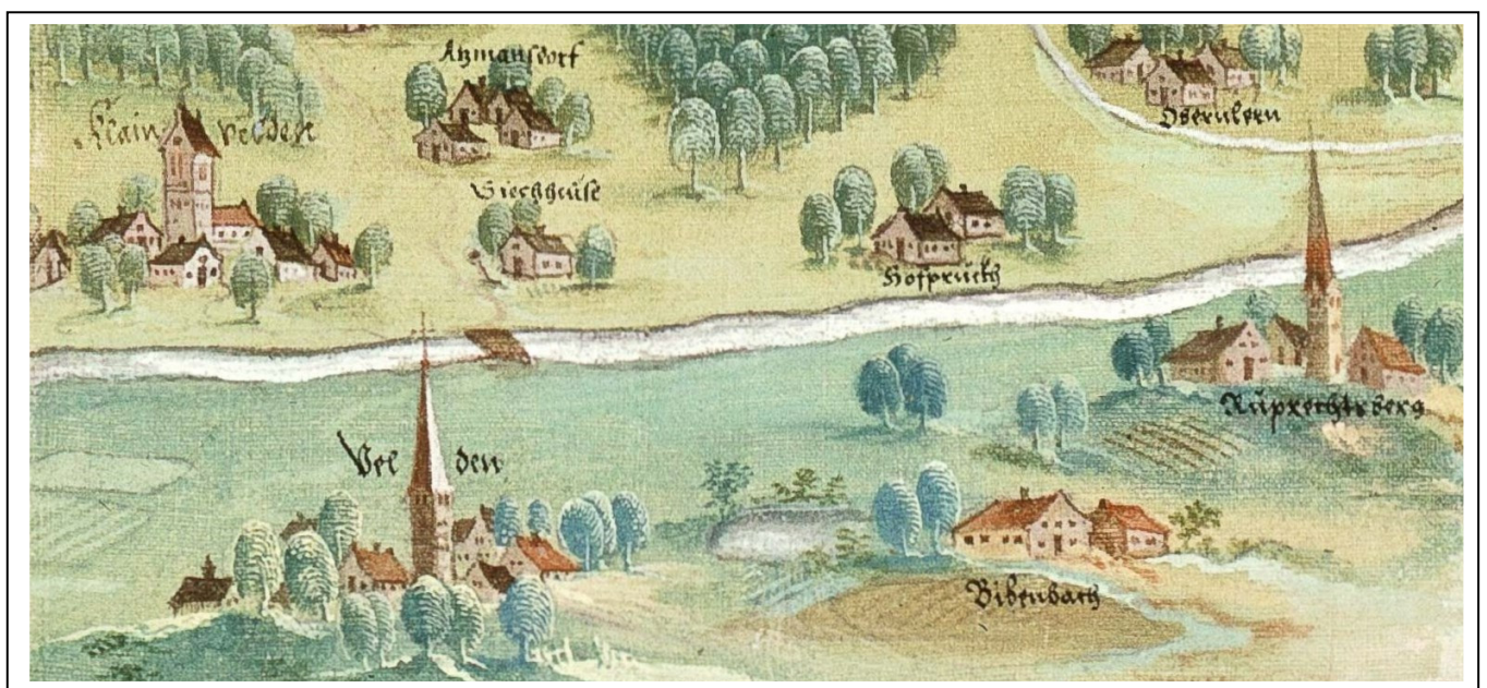
Auszug aus der Wildbannkarte der Reichsherrschaft Fraunhofen. Der Regensburger Maler Hieronymus Van de Venne hat 1584 diese „Wildbanngranzkarte“ gefertigt. - Links oben: Kleinvelden mit Kirche. Rechts: Ruprechtsberg . - Unten links: Velden ; mitte Biedenbach .
